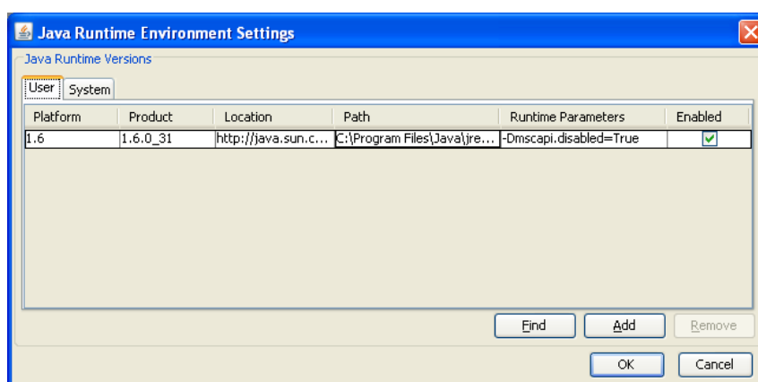
Figura 3.12. Desabilitando a camada MSCAPI (-Dmscapi.disabled=true)
